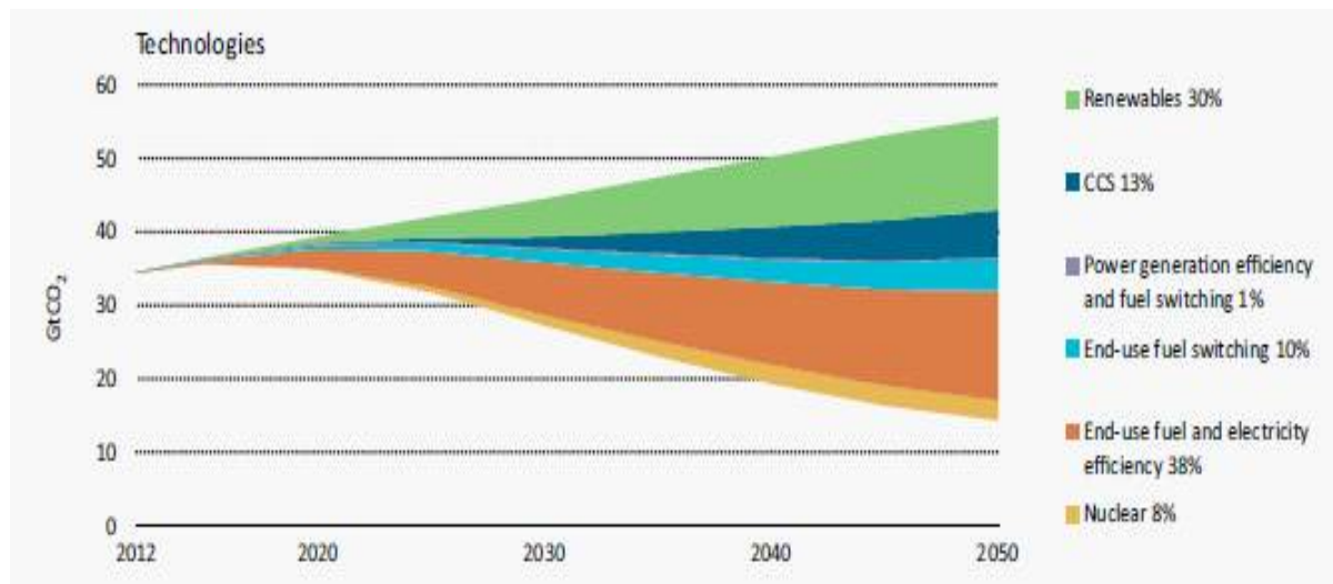
[그림 7] 2050년까지의 에너지부문 장기 감축수단별 이산화탄소 감축량
