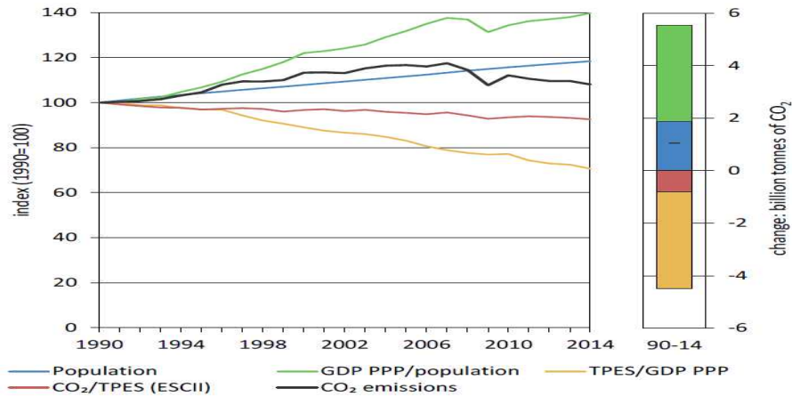
[그림 1] OECD의 탈동조화 추이
